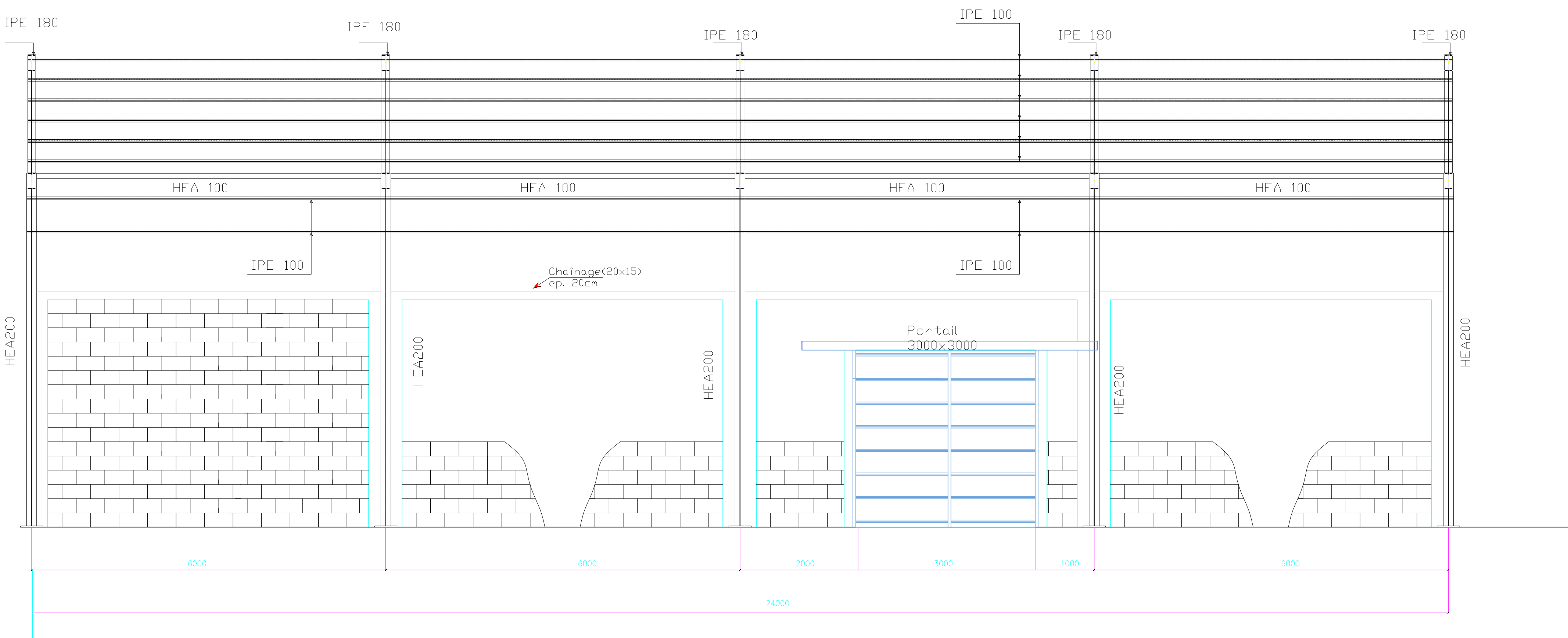
VUE FAÇADE LATÉRALE GAUCHE
